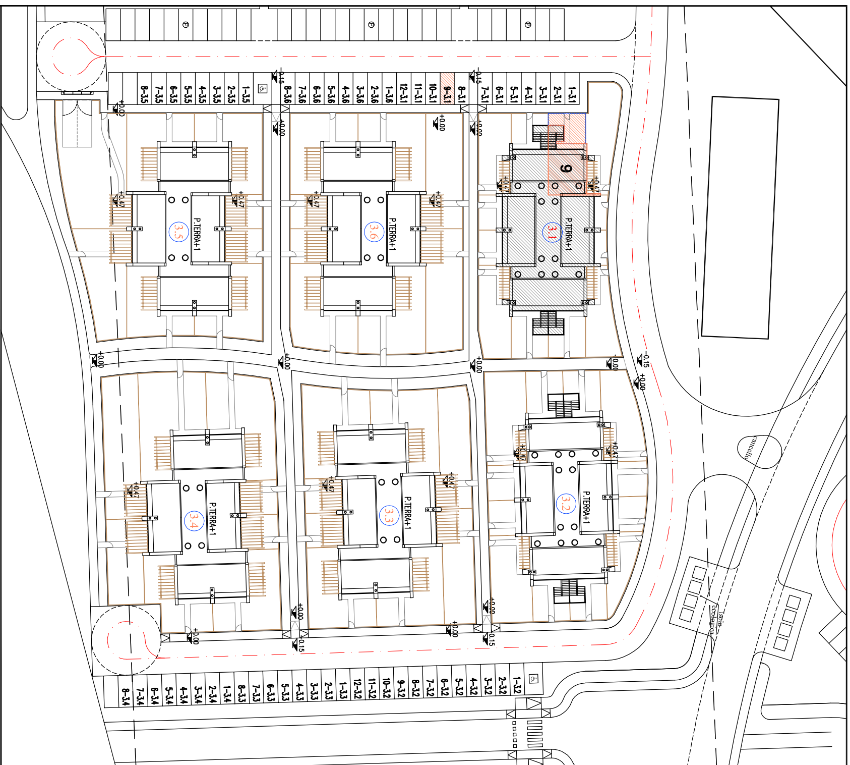
PIANO TERRA - scala 1:100
