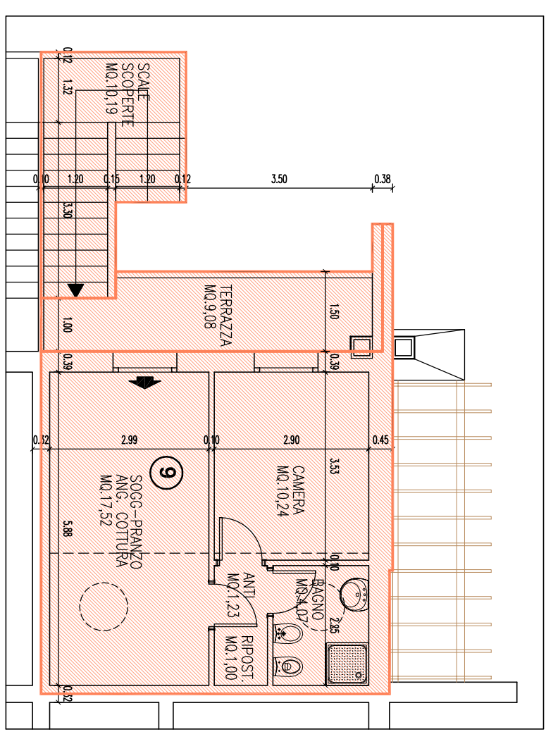
PIANO PRIMO - scala 1:100
